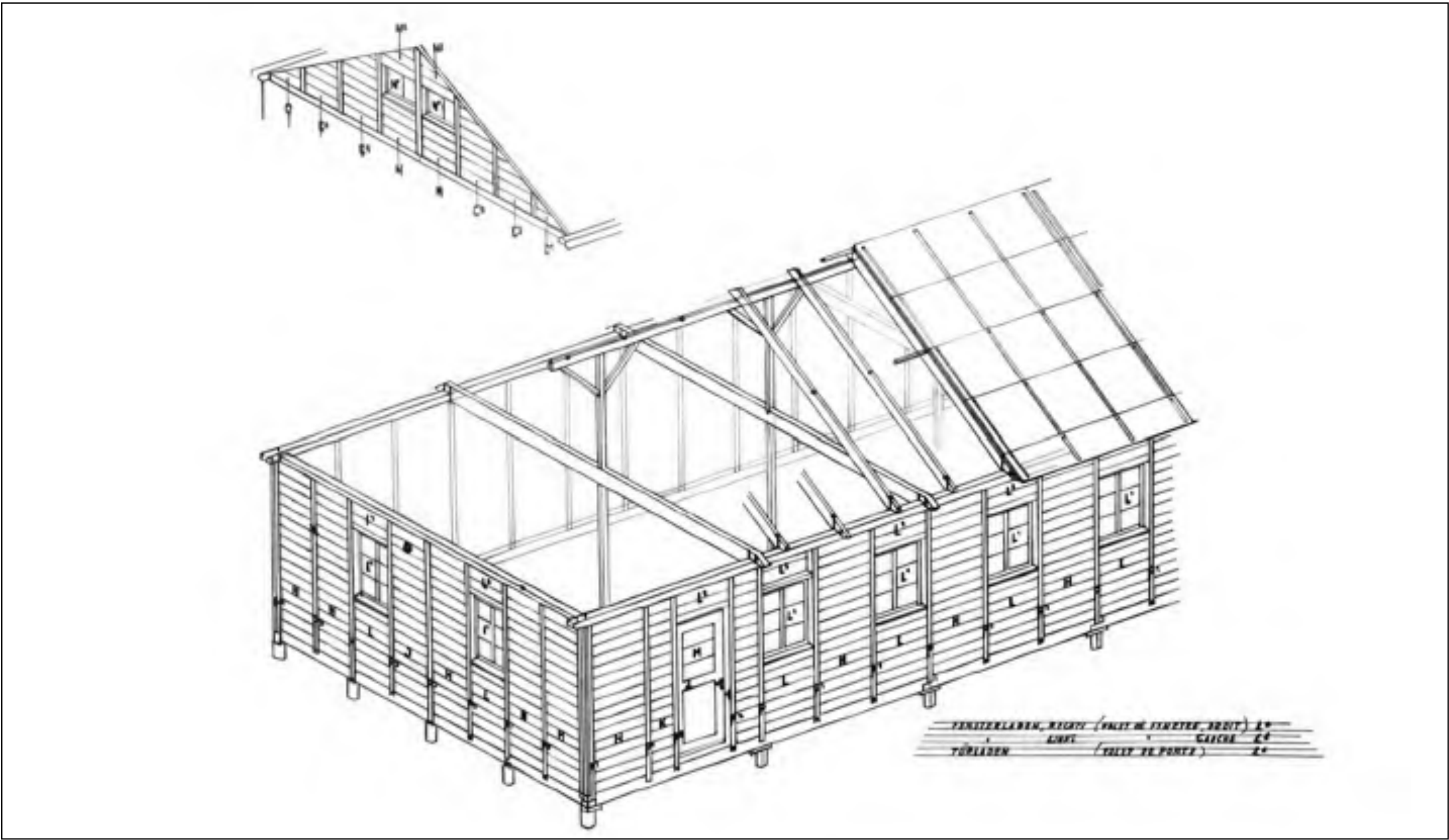
Cronbaracke Isometrie der Holzkonstruktion Archiv Jean Cron AG
