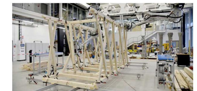
Teilprojekt 7: Auf- und Rückbau Tragkonstruktion >
