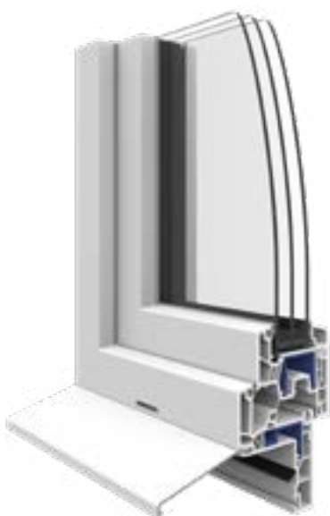
Finestra in PVC Ego®Allround con telaio di ricambio
