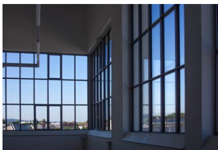
Innenansicht nach der Sanierung mit forster unico XS Industriegebäude Arbomec (unter Denkmalschutz) in Arbon, Schweiz (03_DSC07869)
